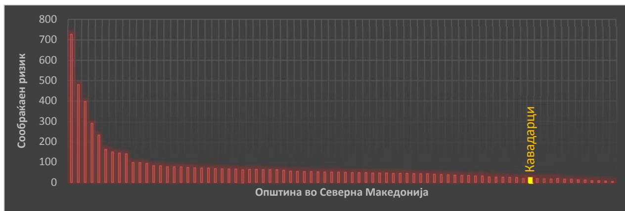
Figure 5 Вредности на сообраќајно пондерираниот ризик од повреда по општини во Република Северна Македонија, 2021 година 8
