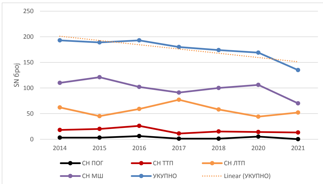
Figure 3 Бројот на сообраќајни незгоди на територијата на општина Кавадарци во периодот од 2014 до 2021 година
