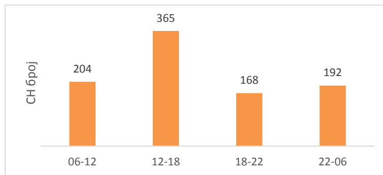
Графикон 12 _ Часовна распределба на вкупниот број сообраќајни незгоди на територијата на општина Кавадарци во периодот од 2014 до 2018 година
