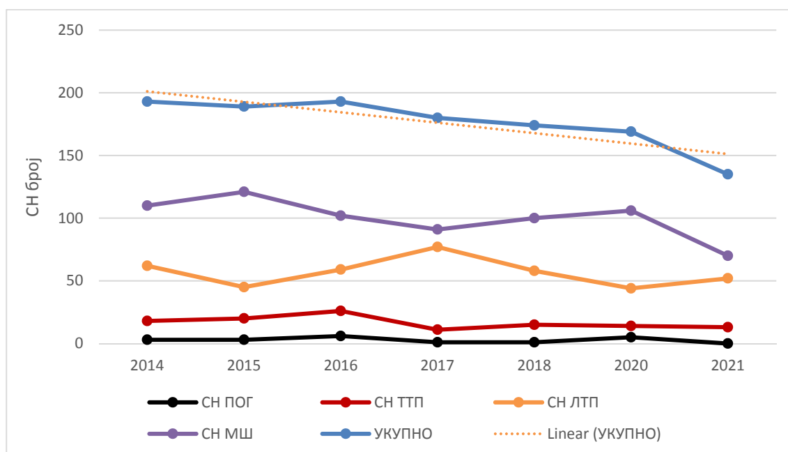
Графикон 2 _ Број на сообраќајни незгоди на подрачјето на општина Кавадарци
