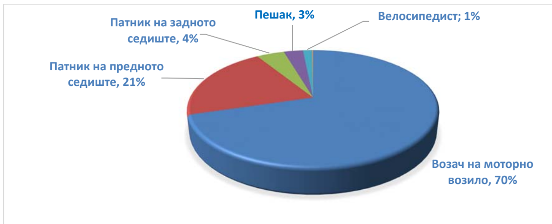
Figure 7 Распределба на повредени учесници според природата на учество во сообраќајот, општина Кавадарци, во периодот од 2020. до 2021. година
