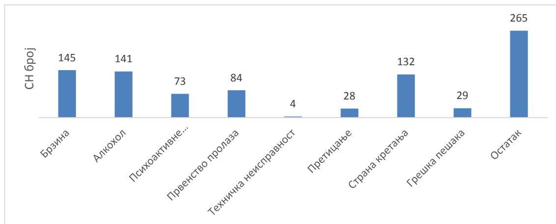
Графикон 10 _Причини за сообраќајни незгоди на подрачјето на општина Кавадарци во периодот од 2014 до 2018 година
