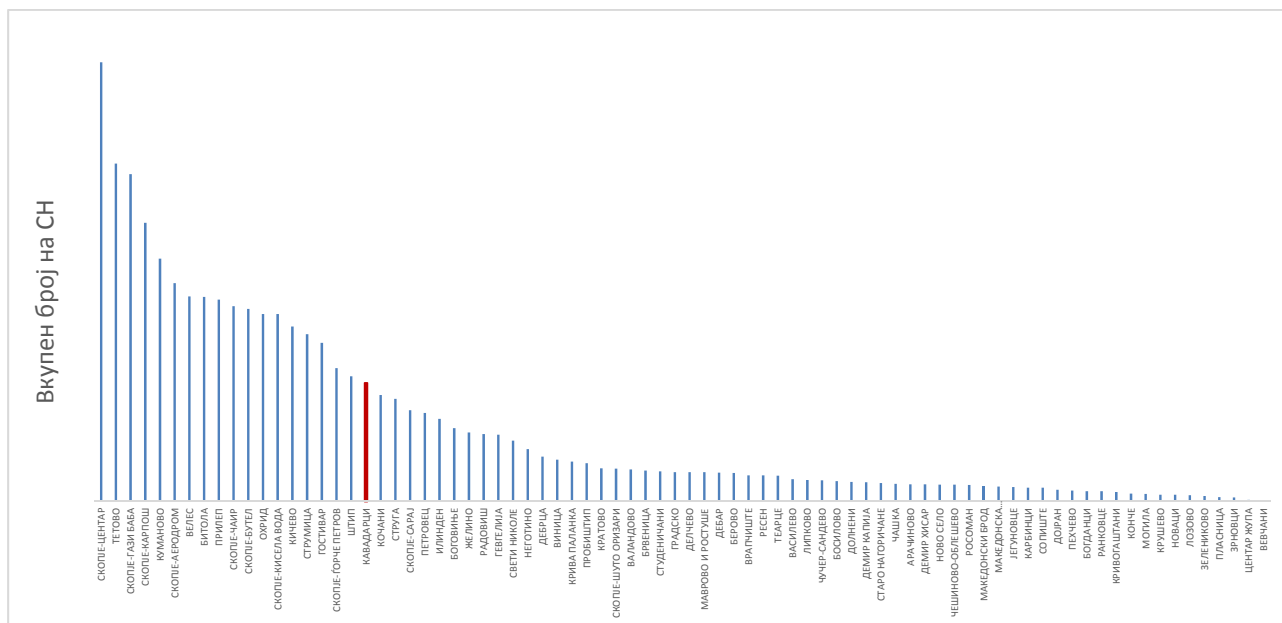
Графикон 1 _Распределба на општините во однос на вкупниот број на сообраќајни незгоди во периодот од 2020 до 2021 година
