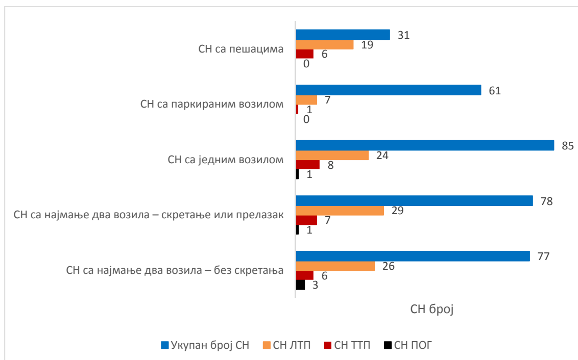
Графикон 9 _ Распределба на сообраќајни незгоди по видови на незгода на територијата на општина Кавадарци во периодот од 2020 до 2021 година
