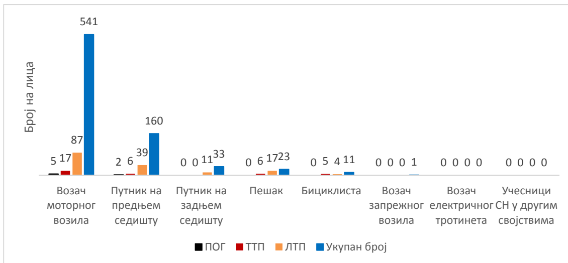
Графикон 7 _Распределба на лица кои учествувале во сообраќајни незгоди според природата на учеството во сообраќајот, како и последиците на територијата на општина Кавадарци во периодот од 2020 до 2021 година
