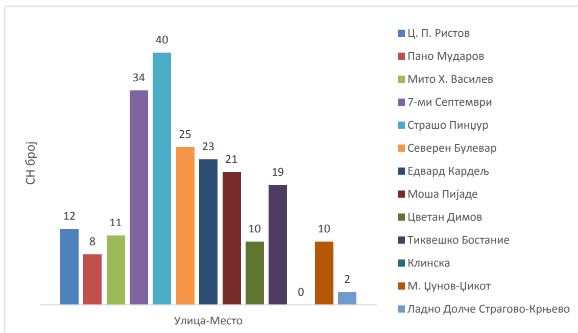
Графикон 15 _Распределба на сообраќајни незгоди во однос на улица-место на настанување на територијата на општина Кавадарци во периодот од 2018 до 2022 година
