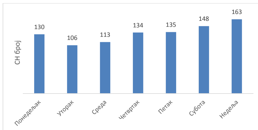
Графикон 11 _ Распределба на сообраќајни незгоди по денови во неделата на подрачјето на општина Кавадарци во периодот од 2014 до 2018 година
