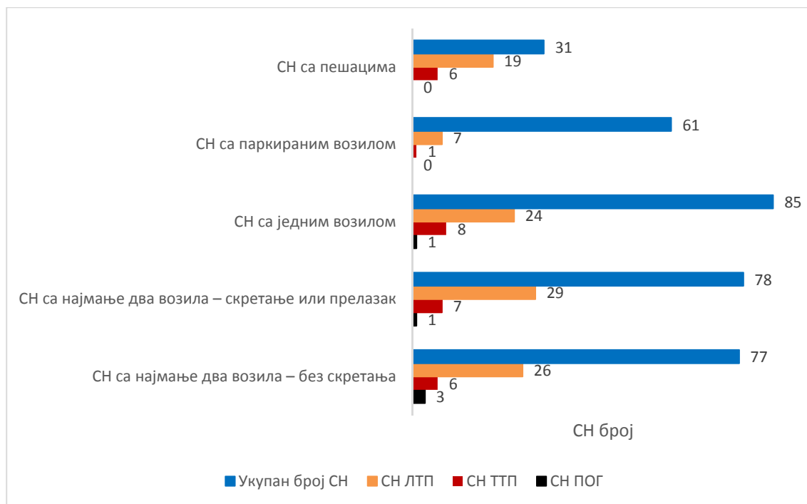
Figure 8 Распределба на жртвите кои учествувале во сообраќајни незгоди според видот на несреќата на територијата на општина Кавадарци, што се случила на локалниот пат, улица и булевар, во периодот од 2020. до 2021. година
