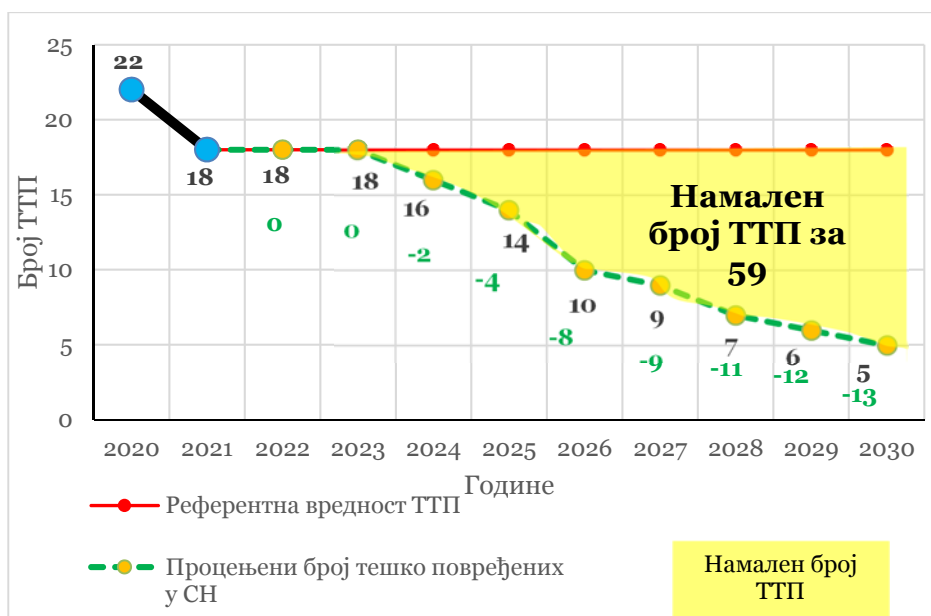
Figure 10 Проценка на бројот на тешко повредени лица и постигнување на целта за намалување на бројот на тешко повредени лица
