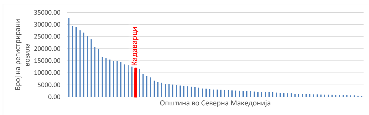
Figure 2 Позицијата на општина Кавадарци според бројот на регистрирани возила, во однос на другите општини во Република Северна Македонија 2
