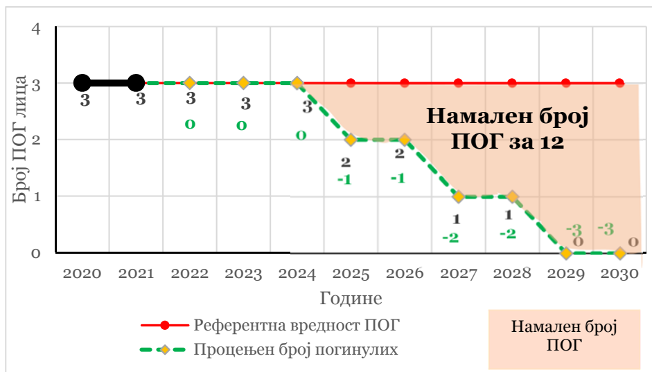
Figure 9 Проценка на бројот на загинали и постигнување на целта за намалување на бројот на жртви
