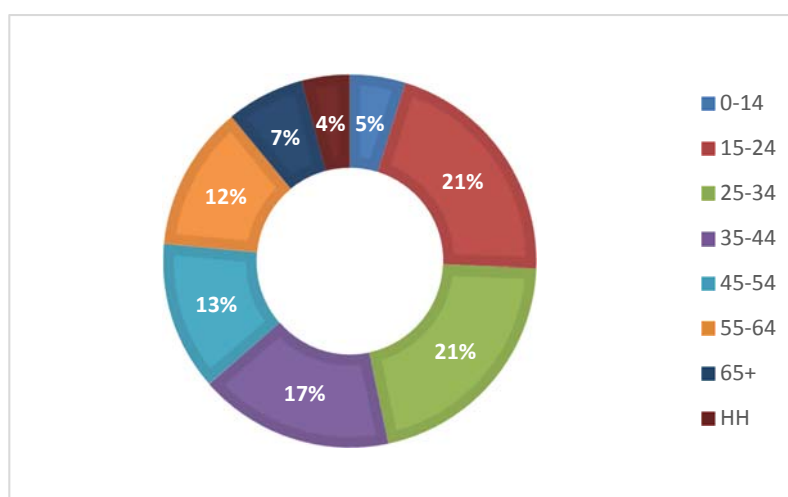
Figure 6 Распределба на жртвите кои учествувале во сообраќајни незгоди според возрасни категории, на територијата на општина Кавадарци во периодот од 2020 до 2021 година
