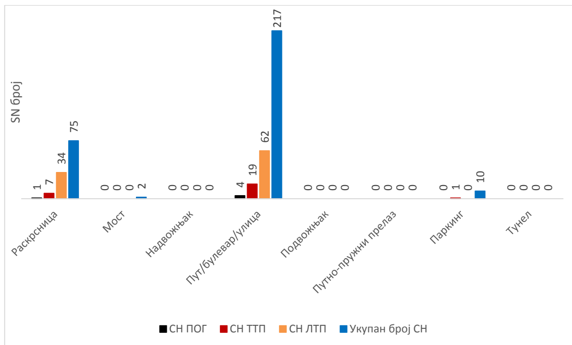
Графикон 14 _Распределба на сообраќајни незгоди во однос на конкретното место на случување на територијата на општина Кавадарци во периодот од 2020 до 2021 година
