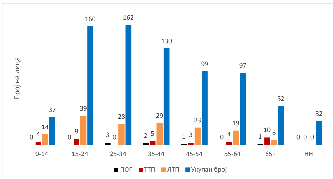
Графикон 5 _ Распределба на лица кои учествувале во сообраќајни незгоди во зависност од старосната структура на лицата, како и последиците на територијата на општина Кавадарци во периодот од 2020 до 2021 година
