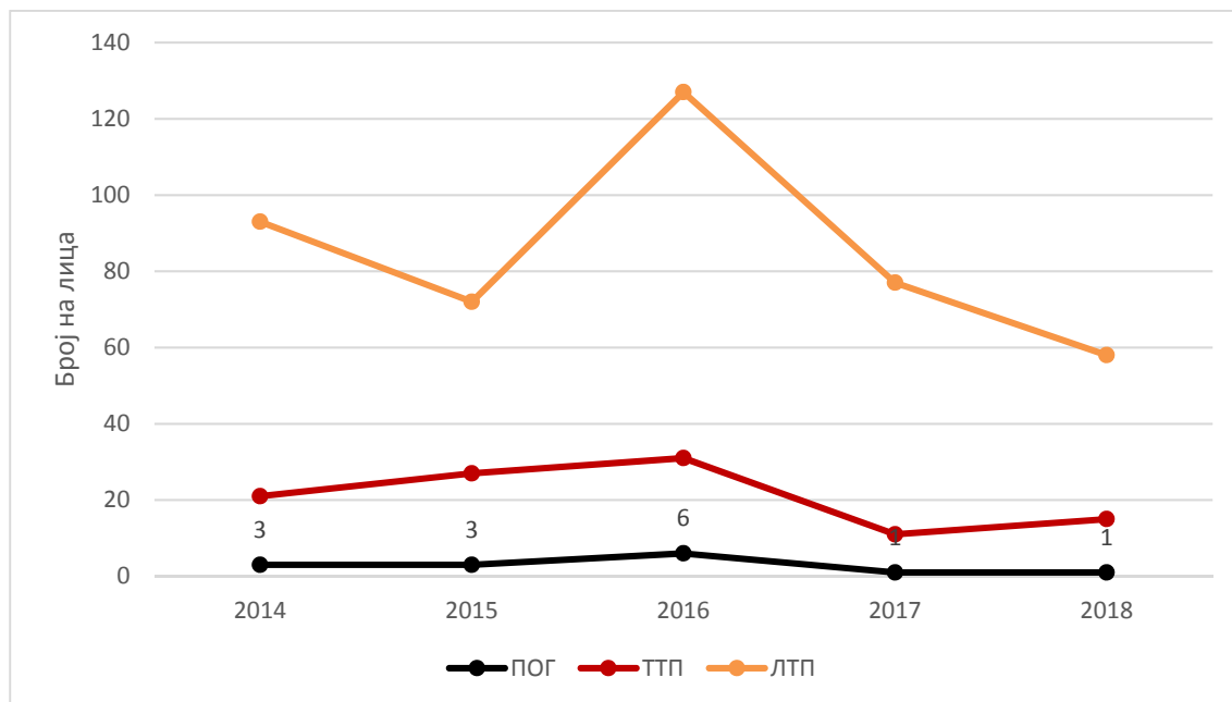
Графикон 3 _ Бројот на жртви на територијата на општина Кавадарци во периодот од 2014 до 2018 година
