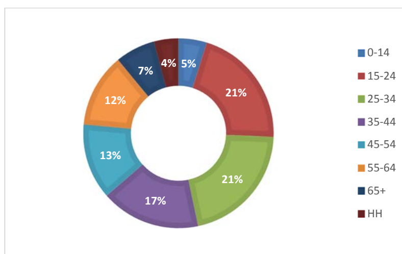
Графикон 4 _ Распределба на лица кои учествувале во сообраќајни незгоди во зависност од старосната структура на лицата на територијата на општина Кавадарци во периодот од 2020 до 2021 година
